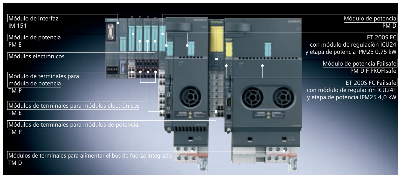
Configuración de una estación ET 200S con convertidores de frecuencia
